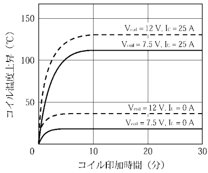
コイル温度上昇
